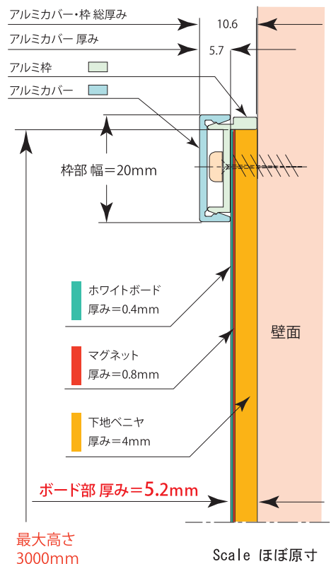
タイプ A 縦断面図
