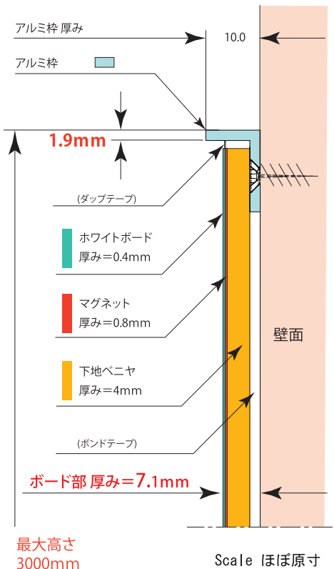
タイプ L 縦断面図
